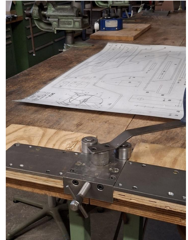
Rollbieger BSAÖ & Plan M 1:1 Roll Bender VSAÖ & Plan Scale 1:1
